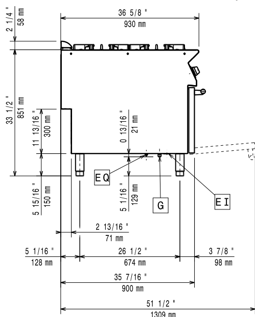
Zij aanzicht
